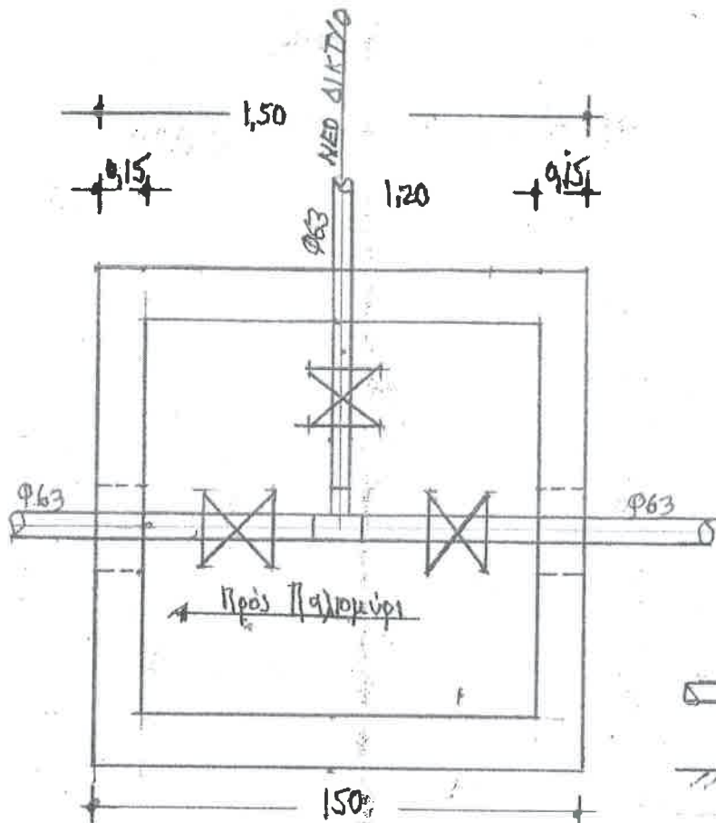
ΚΑΤΩΨΗ ΦΡΕΑΤΙΟΥ ΣΤΗΝ Δ0
