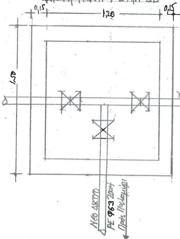
ΚΑΤΩΨΗ ΦΡΕΑΤΙΟΥ ΣΤΗΝ Δ15
