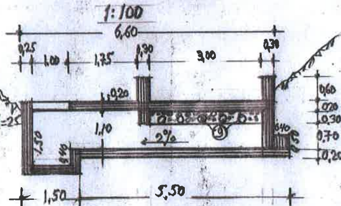
ΤΟΜΗ Δ-Δ 1:100
