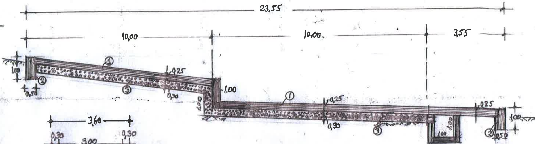
ΤΟΜΗ Γ-Γ 1:100
