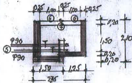
ΤΟΜΗ Ε-Ε 1:100
