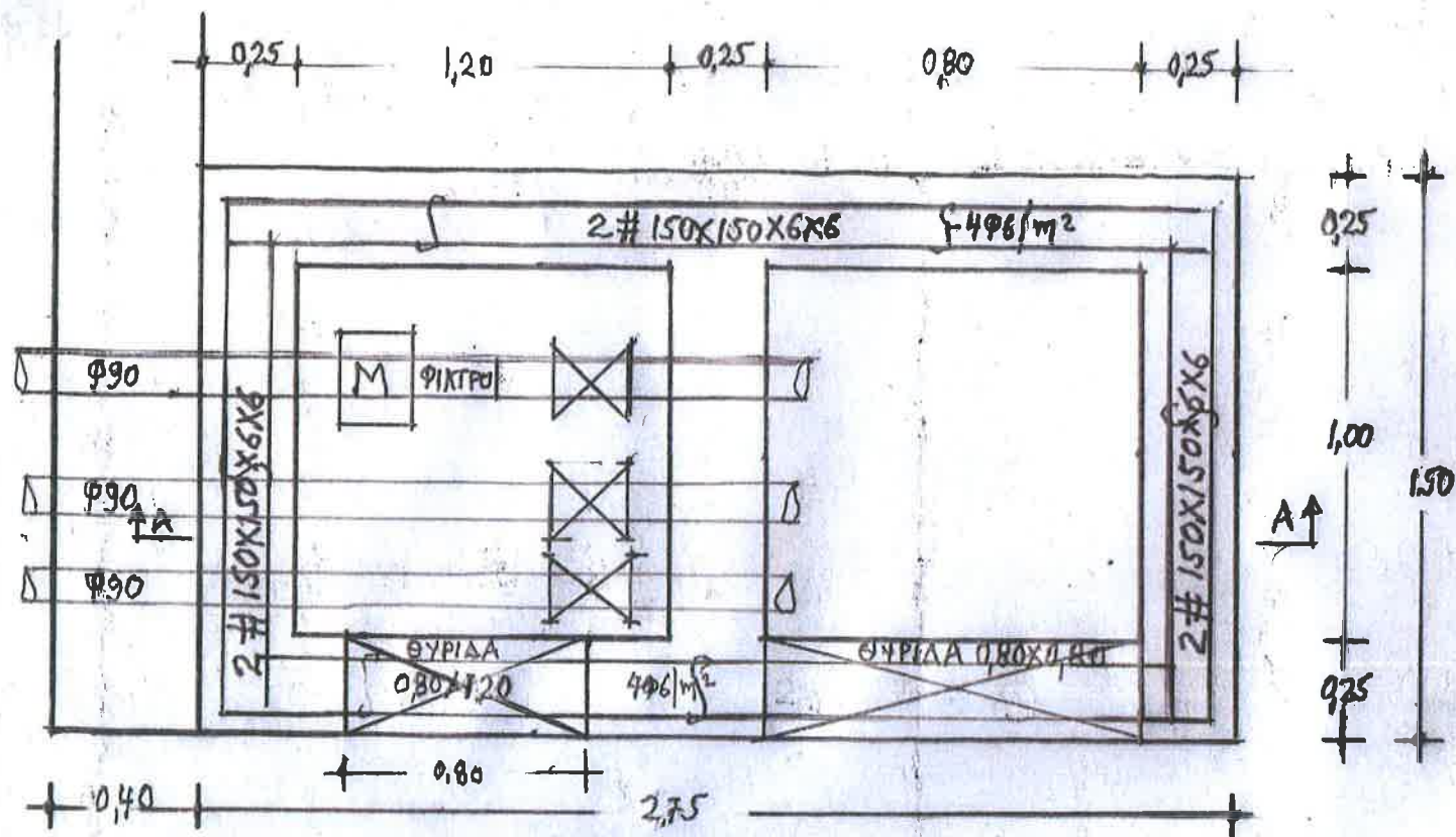
ΚΑΤΟΨΗ ΦΡΕΑΤΙΟΥ 1:20
