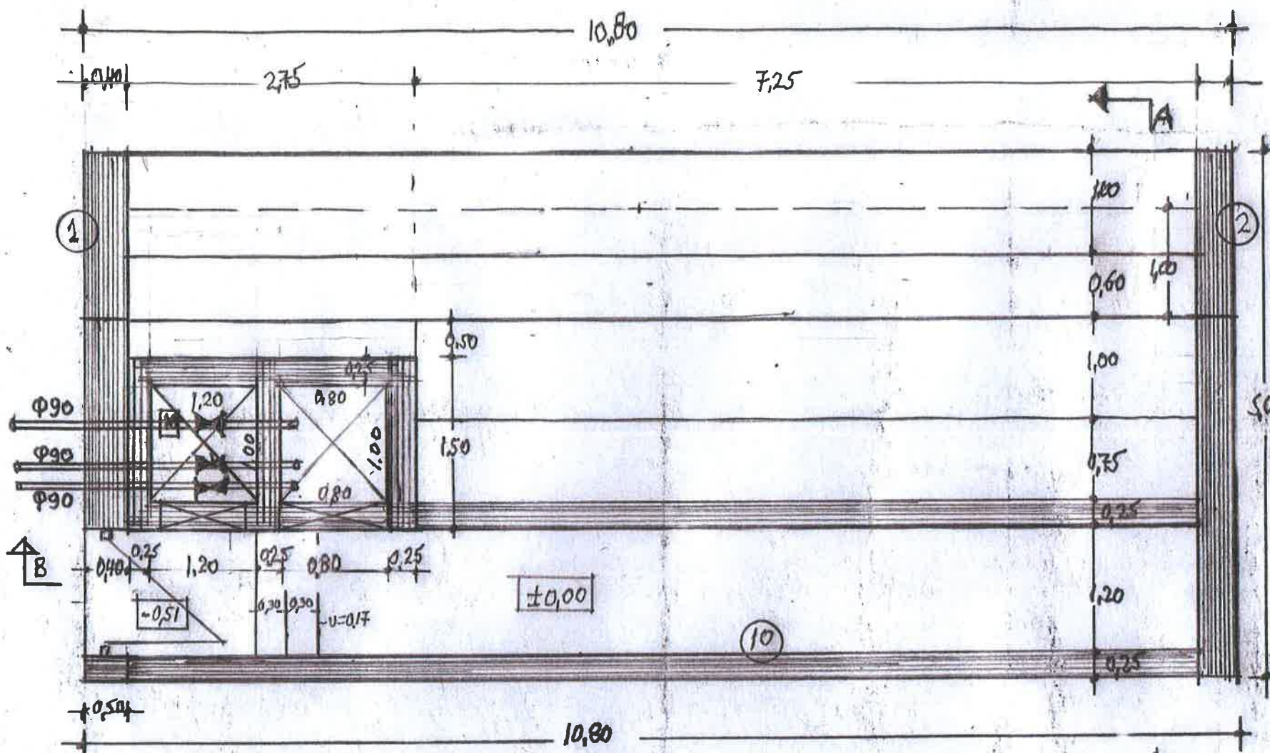
ΟΡΙΖΟΝΤΙΟΓΡΑΦΙΑ ΥΔΡΟΜΑΣΤΕΥΣΗΣ 1:50
